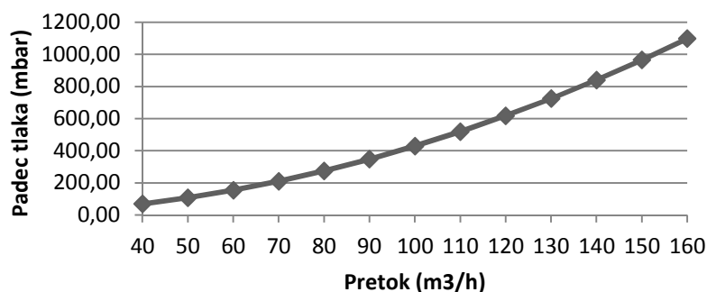
Pretočne karakteristike DN80
